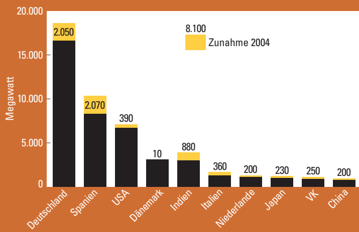
Abbildung 6. Installierte Windkraftleistung in den zehn führenden Ländern - 2004
