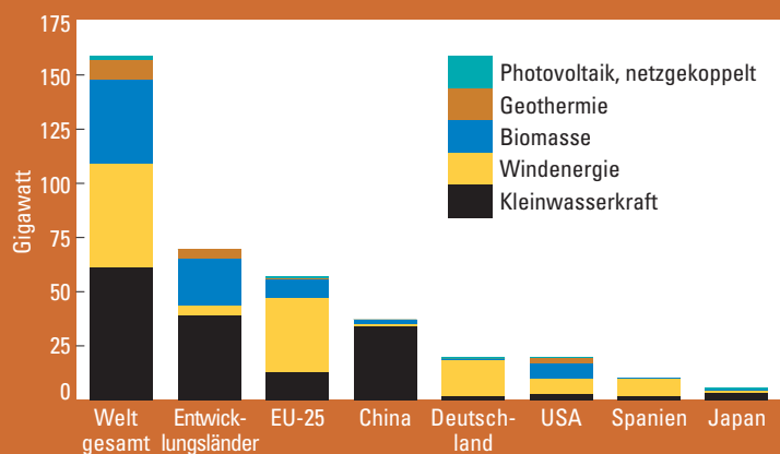
Abbildung 5. Kapazitäten zur Erzeugung von Regenerativstrom in den fünf führenden Ländern, der EU und der Dritten Welt - 2004
