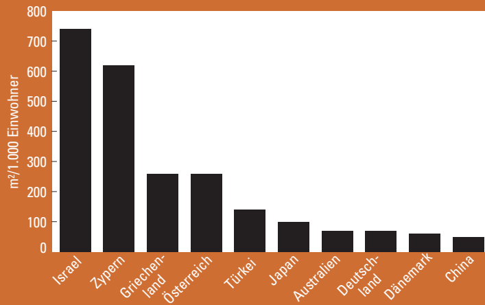
Abbildung 8. Installierte Anlagen zur solaren Warmwasserbereitung je tausend Einwohner
