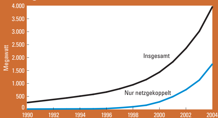
Abbildung 3. Photovoltaik, weltweit installierte Leistung - 1990-2004
