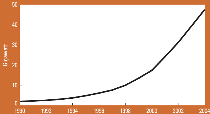
Abbildung 4. Windkraft, weltweit installierte Leistung - 1990-2004
